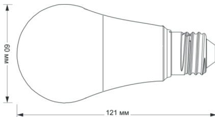
Рисунок 1 – Габаритные размеры.
