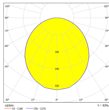
Опал 120°
