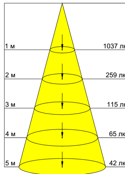
Опал 120°
