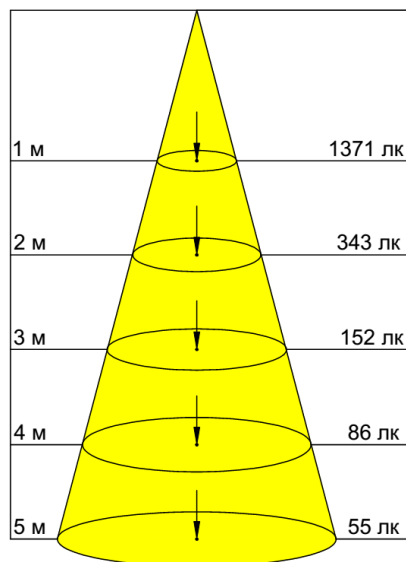
Микропризма 90°
