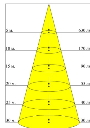
Geniled Колокол 200W 45°
